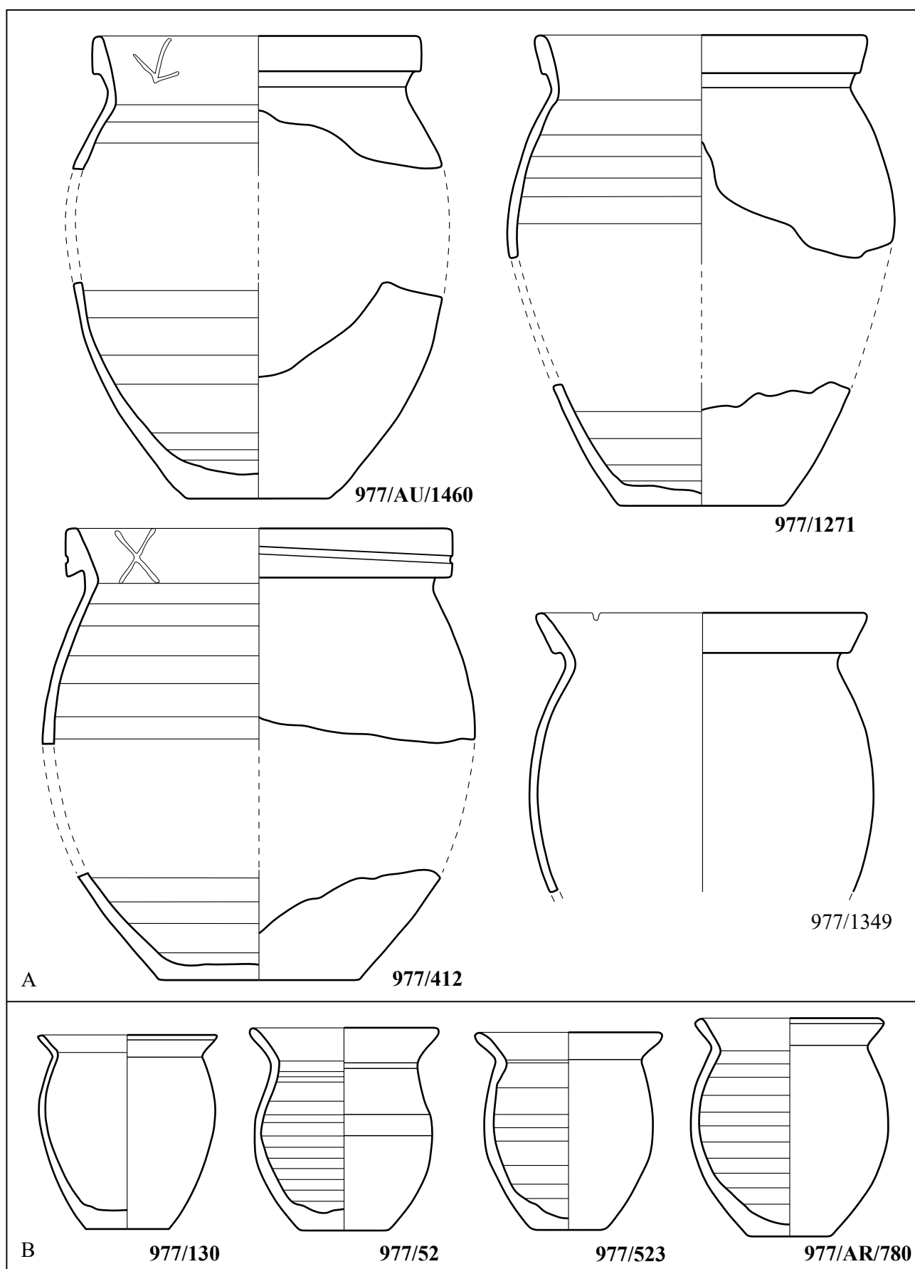
Ceramica in impasto grezzo di epoca ellenistica. A. Olle ovoidi con orlo a fascia piatta (A.I.1.4). B. Olle e ollette ovoidi a pareti di spessore ridotto (0,3-0,4 cm) con orlo semplice arrotondato o a finta fascia (A.I.1.5). Scala 1:2.
