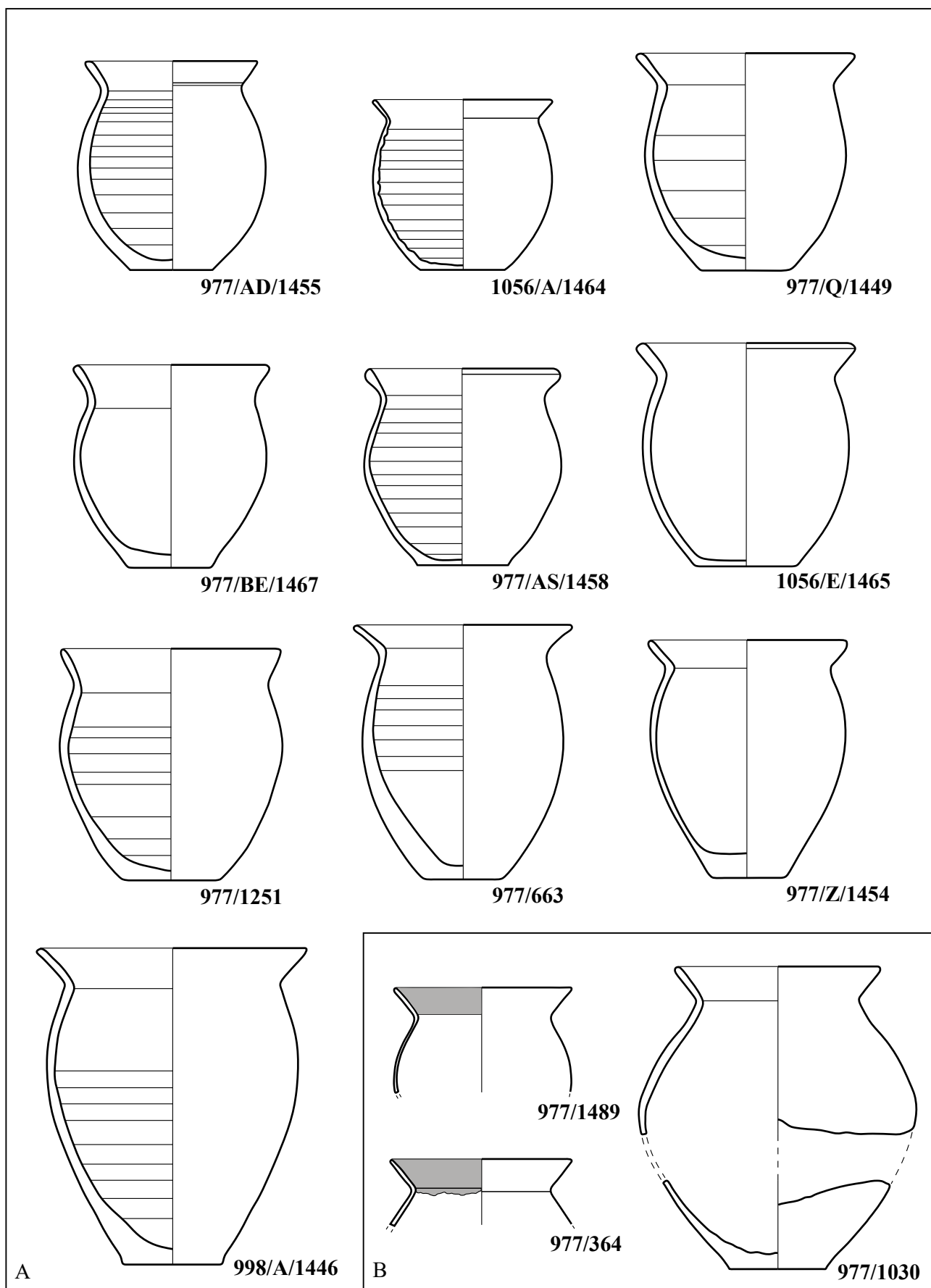
Ceramica in impasto grezzo di epoca ellenistica. A. Olle e ollette ovoidi a pareti di spessore ridotto (0,3-0,4 cm) con orlo semplice arrotondato o a finta fascia (A.I.1.5). B. Olle e ollette ovoidi a pareti di spessore ridotto (0,2-0,3 cm) con orlo semplice arrotondato o a finta fascia, leggermente più grandi delle precedenti e dal corpo più tondeggiante, quasi globulare (A.I.1.6). Scala 1:2.
