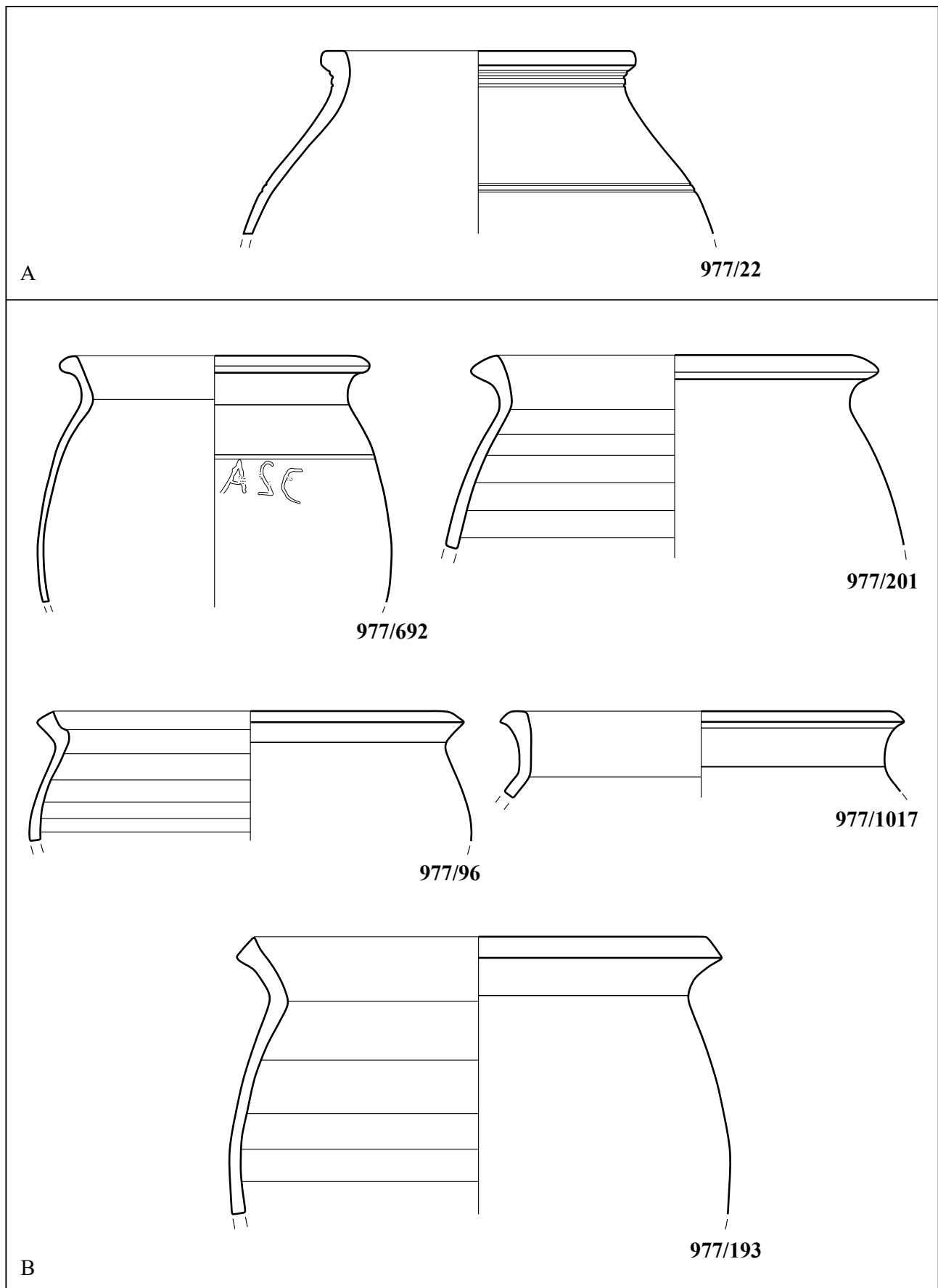
Ceramica in impasto grezzo di epoca ellenistica. A. Olle ovoidi con orlo modanato senza collo (A.I.1.7). B. Olle ovoidi con orlo a sezione triangolare (A.I.1.8). Scala 1:2.
