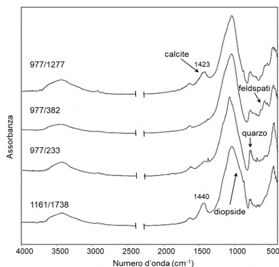
Fig. 2. Spettri FTIR acquisiti su pastiglie in bromuro di potassio delle polveri dei quattro campioni di ceramica di impasto dal pozzo studiati per la temperatura di cottura. Sono indicate le bande caratterizzanti delle principali fasi cristalline. Per la calcite si riporta altresì il numero d'onda del massimo della banda compresa tra 1450 e 1420\text{ cm}^{-1} , poiché esso risulta indicativo per stabilire se la fase in questione è primaria oppure riformata (si veda il testo). La banda più intensa, situata tra 1100 e 1000\text{ cm}^{-1} , è dovuta agli stiramenti dei legami Si-O di tutte le componenti silicatiche, ivi compresa la matrice amorfa, dei materiali ceramici.
