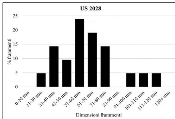
Grafico 5. Il grafico mostra la percentuale del numero dei frammenti ossei suddivisi in gruppi dimensionali per l'US 2028.
