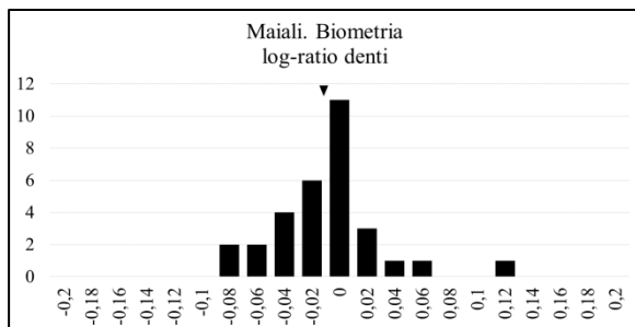
Grafico 19. Maiali. Log-ratio dei denti.
