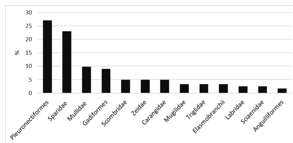
Grafico 23. Distribuzione dei taxa identificati (NR 122), vedi Tab. 14 per relative identificazioni di specie.
