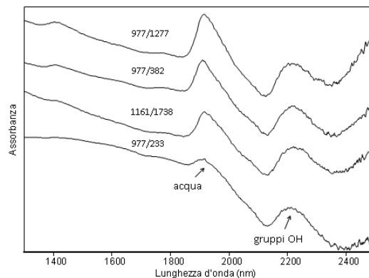
Fig. 1. Spettri in riflessione diffusa nel vicino IR dei quattro campioni di ceramica di impasto dal pozzo studiati per la temperatura di cottura.
