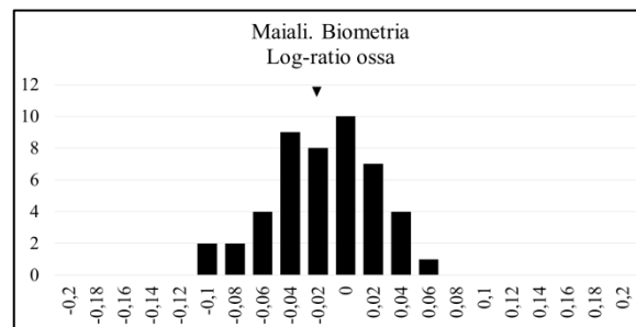
Grafico 20. Maiali. Log-ratio delle ossa. Si sono usate solo le misure delle ossa fuse.
