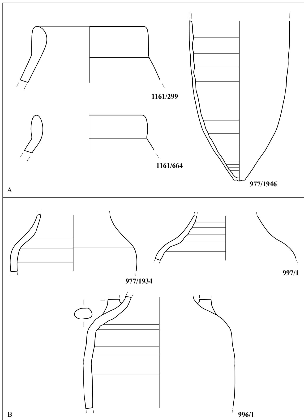
Anfore. A. Puniche. B. Greco-italiche. Scala 1:4; 1161/299, 1161/664: scala 1:2.
