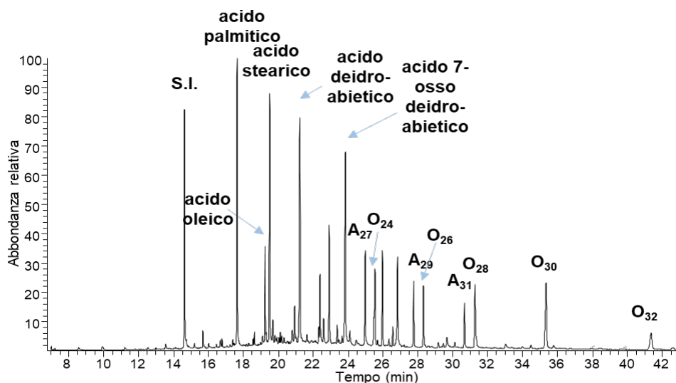
Fig. 3. Cromatogramma ottenuto dall'analisi GC-MS dell'estratto lipidico dell'anfora 977/1950 . Legenda: A_n = idrocarburo saturo a catena lineare a n atomi di carbonio; O_n = alcol a catena lineare a n atomi di carbonio; S.I. = standard interno.
