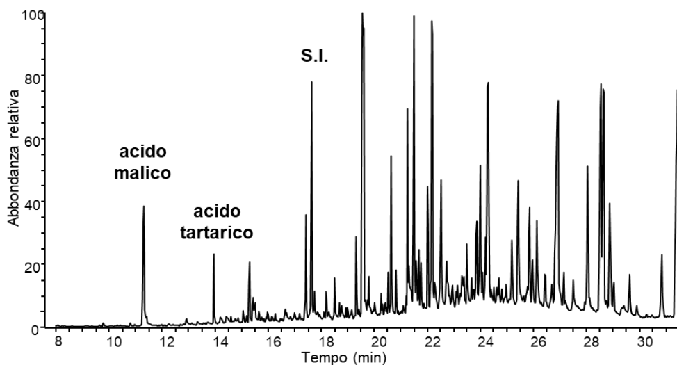
Fig. 4. Cromatogramma ottenuto dall'analisi GC-MS dell'estratto in metanolo acidificato dell'anfora 977/1950 . Legenda: S.I. = standard interno.
