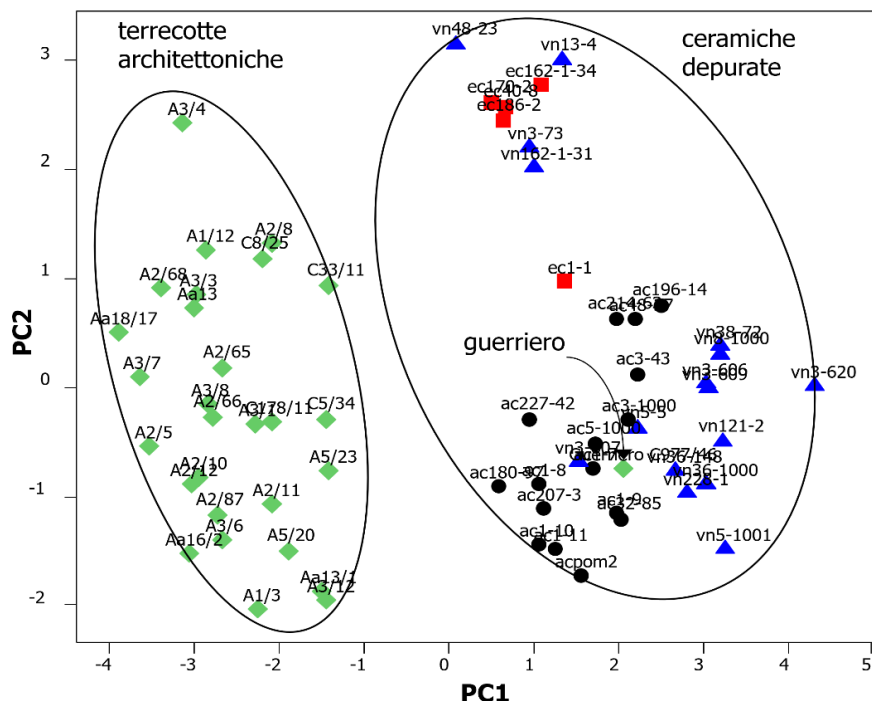
Grafico 2. Grafico degli scores ottenuto dall'analisi delle componenti principali dei dati di composizione elementare del fregio raffigurante il guerriero 977/46, di un insieme di terrecotte architettoniche e di ceramiche depurate di produzione tarquiniese.
