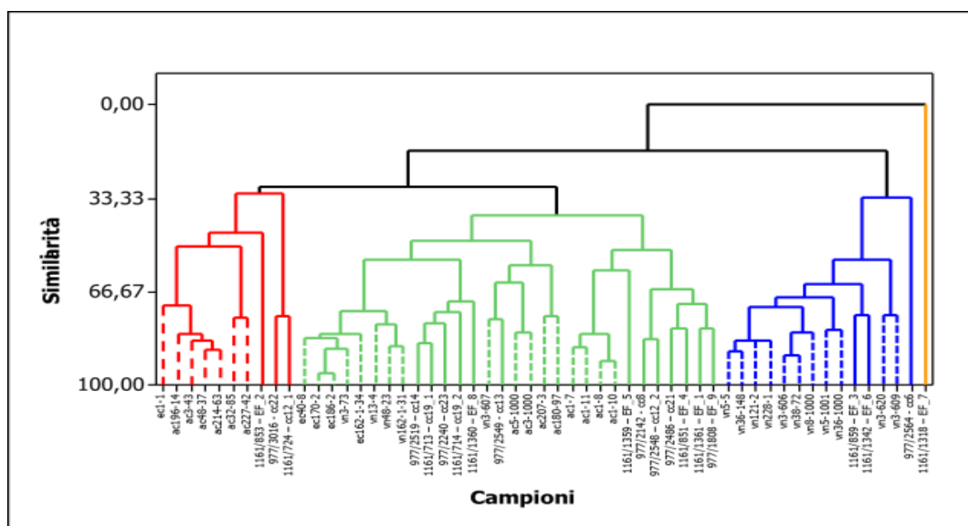
Grafico 1. Dendrogramma ottenuto dall'analisi dei cluster dei dati di composizione elementare delle ceramiche etrusche figurate e a vernice nera ellenistica dal pozzo (linee verticali continue) poste a confronto con l'insieme della produzione tarquiniese rappresentata da ceramica acroma, etrusco corinzia e a vernice nera arcaica (linee verticali tratteggiate).
