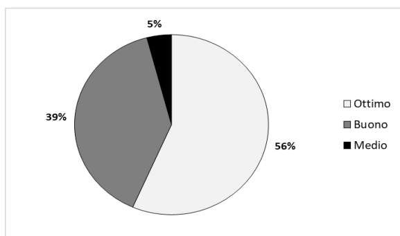
Grafico 21. Grado di conservazione dei reperti rinvenuti nel pozzo (NR 122).
